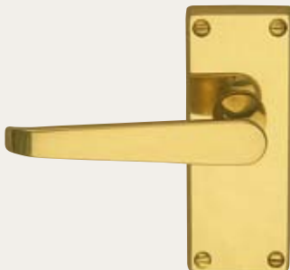
8008 Latch 118×43mm
